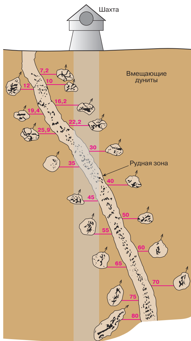
Рис. 4. Геологический разрез до глубины 80 м и по горизонтные планы через рудную зону платинового месторождения “Господская шахта” в Нижнетагильском массиве. Черным цветом отмечены хромитовые тела, обогащенные платиной
